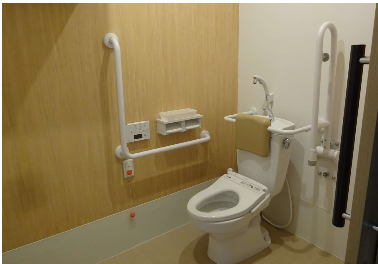
1階の個室トイレの便器中央置きタイプです
